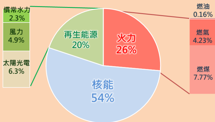
▲ 2020年台灣發電結構 與 2021上半年網路能源聲量結構 圓餅圖
